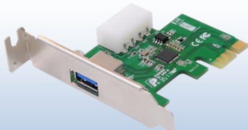
PP1U (1ポートPCIe2.0-USB3.0拡張ボード) x1
