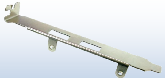
JP0875 (標準PCIブラケット) x1
